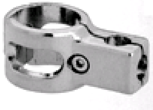
ЈОК53-25 СОЕДИНИТЕЛЬ ОДНОСТОРОННИЙ ТРУБЫ D25 И D10MM
